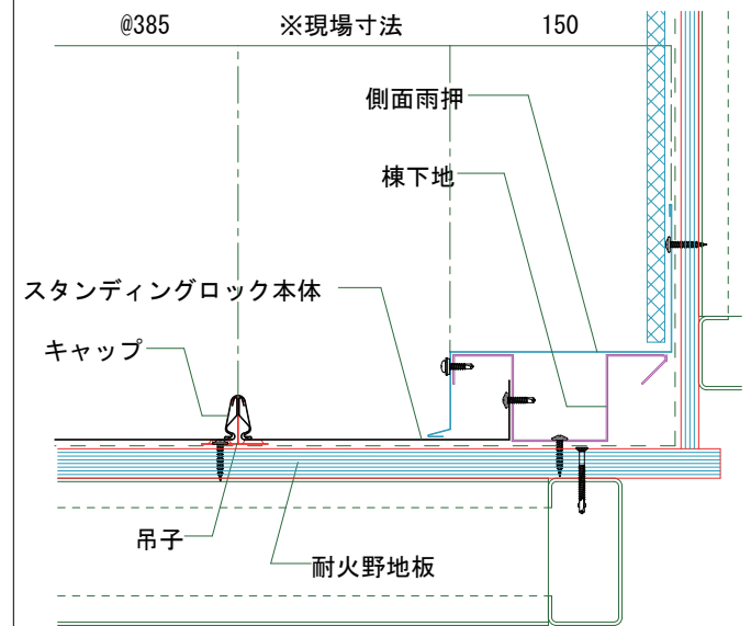
雨押詳細図 (水上側) (鉄骨造下地)
