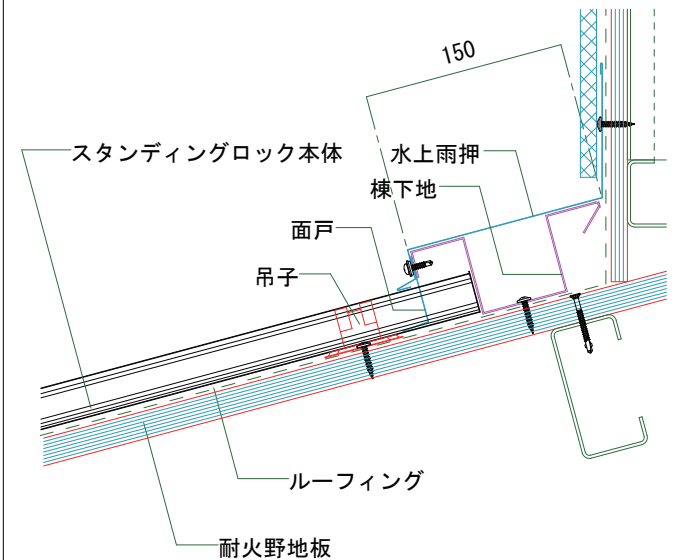
雨押詳細図 (水上側) (鉄骨造下地)
