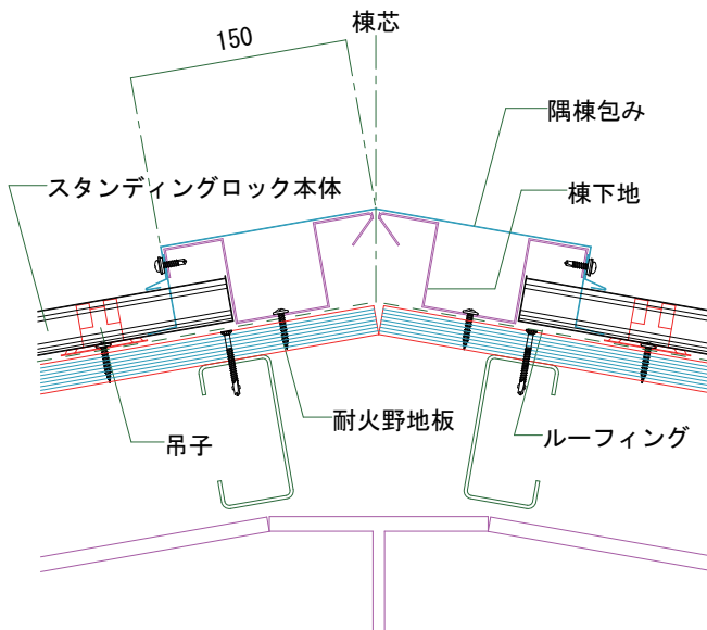
隅棟詳細図 (鉄骨造下地)
