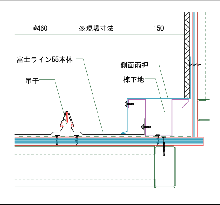
雨押詳細図 (水上側) (鉄骨造下地)
