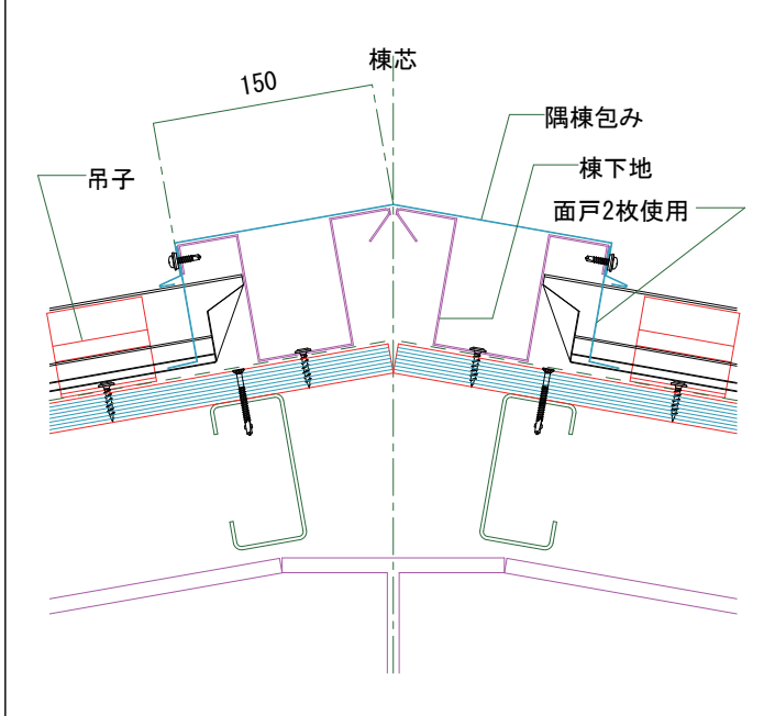
隅棟詳細図 (鉄骨造下地)
