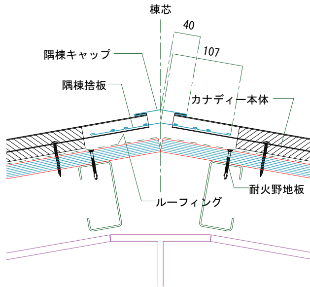
隅棟詳細図 (鉄骨造下地) 断熱材一体型30分耐火認定工法
