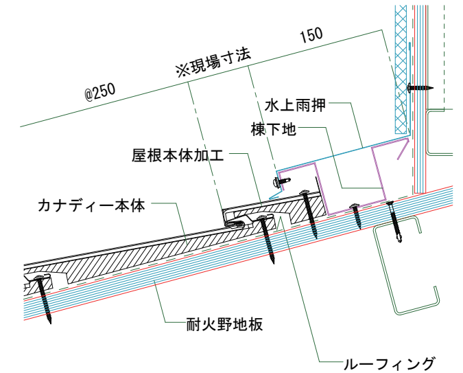
雨押詳細図 (水上側) (鉄骨造下地) 断熱材一体型30分耐火認定工法
