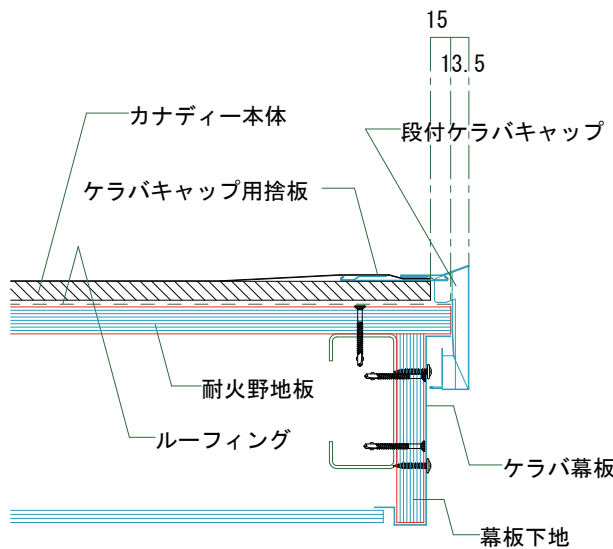
ケラバ詳細図 (鉄骨造下地) 断熱材一体型30分耐火認定工法
