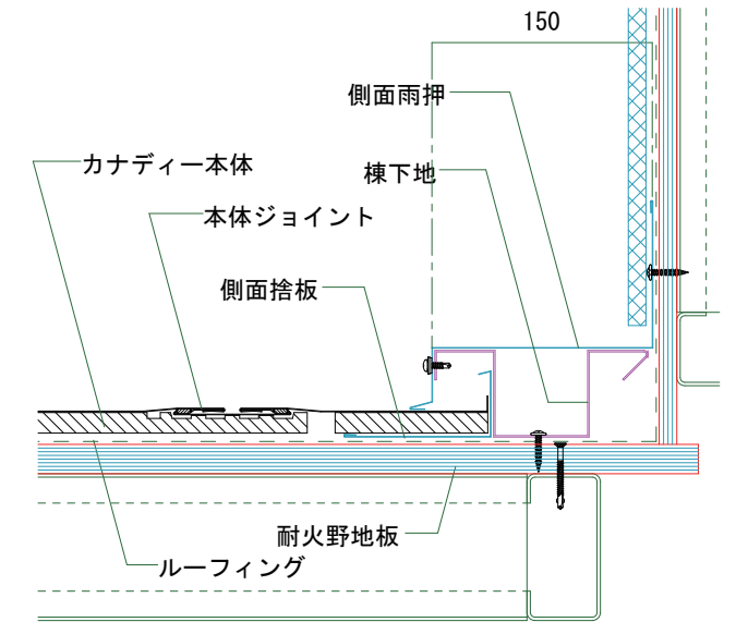
雨押詳細図 (水上側) (鉄骨造下地) 断熱材一体型30分耐火認定工法
